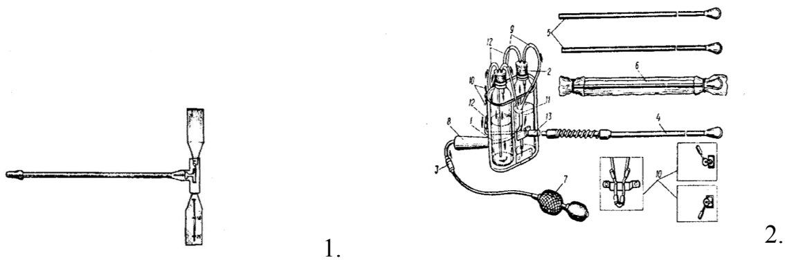
Рис. 38. Прилади для осіменіння свиноматок фракційним способом: 1.- УКП-1, 2.- Уніфікований зонд катетер (УЗК-5): 1- скляні флакони; 2-пробки флаконів; 3- повітряний фільтр; 4- катетер; 5-6 запасні катетери; 7-балон Річардсона; 8-ручка приладу; 9-12 гумова трубка; 10- затискач; 11-сполучний трійник; 13-сполучна муфта.
