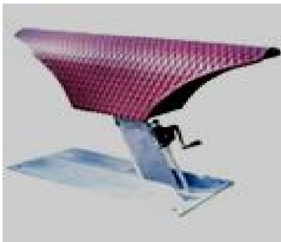
Рис. 21 Фантом для взяття сімені від бугаїв-плідників
