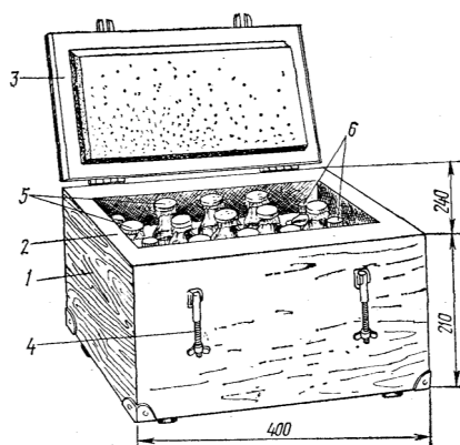
Рис. 35 Термос - ящик для перевезення сперми кнурів-плідників
