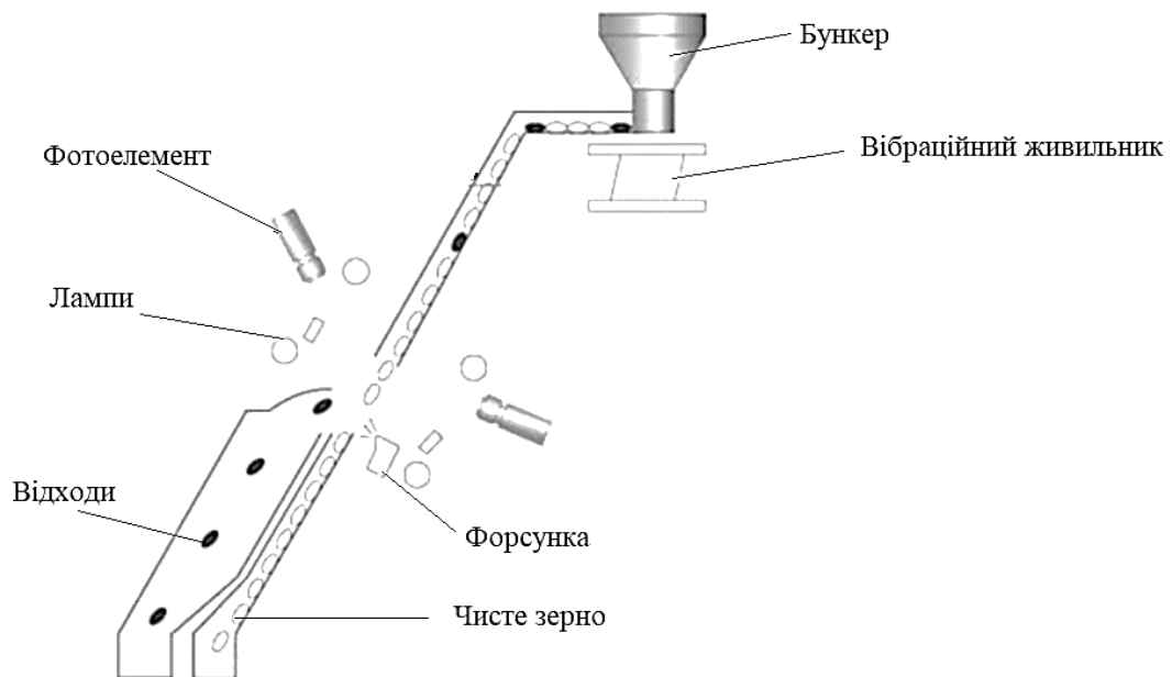
Рис. 4.1 – Принцип роботи фотосепаратора
