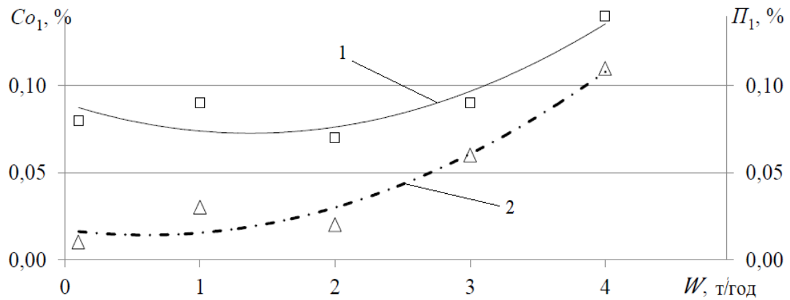
Рис. 3.12 – Залежності вмісту очищених (1) зернівок та домішок (2) у насіннєвій фракції від продуктивності фотосепаратора: C_1 – вміст обрушених зерновок гречки на насіннєвій фракції, %; \Pi_1 – вміст домішок у насінній фракції, %; W – подача оброблюваного матеріалу на скатний лоток фотосепаратора, т/год.
