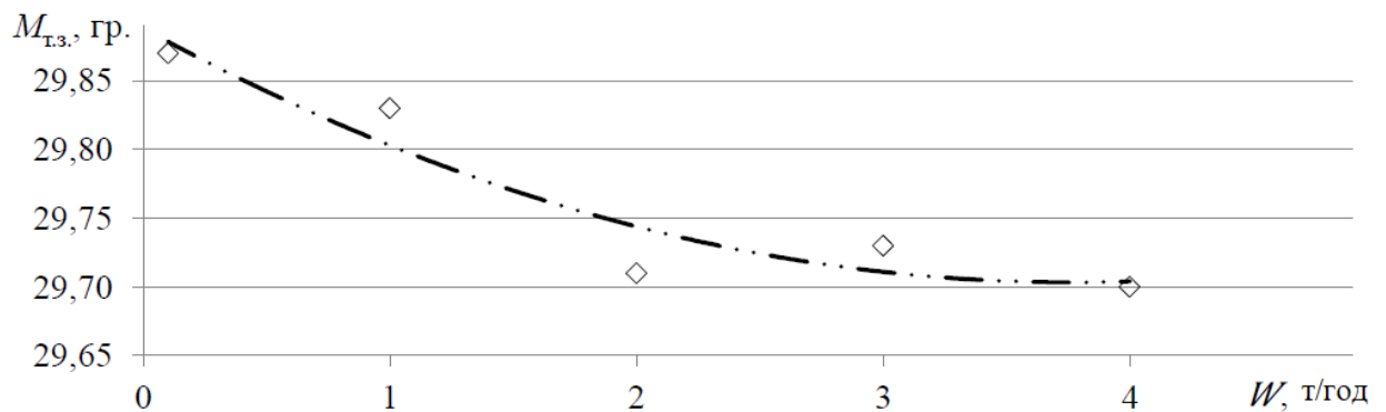
Рис. 3.13 – Зміна маси 1000 зернівок насіннєвої фракції від продуктивності фотосепаратора: M_{т.з.} – маса 1000 зернівок насіннєвої фракції, гр.; W – подача оброблюваного матеріалу на скатний лоток, т/год.
