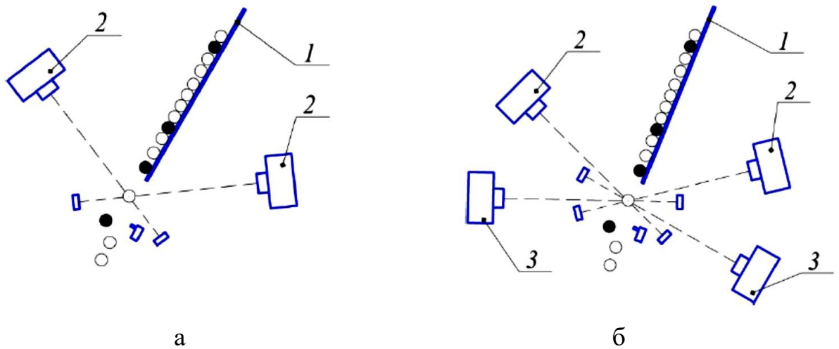
Рис. 3.2 – Схеми оптичного розпізнавання дефектів: а – Схема, що використовується на фотосепараторі Ф10.1; б – схема, яка використовується на фотосепараторі СВ-4; 1 – скатний лоток; 2 – камери, що працюють у видимому діапазоні довжин світлових хвиль; 3 – камери, що працюють у ближньому інфрачервоному діапазоні довжин світлових хвиль
