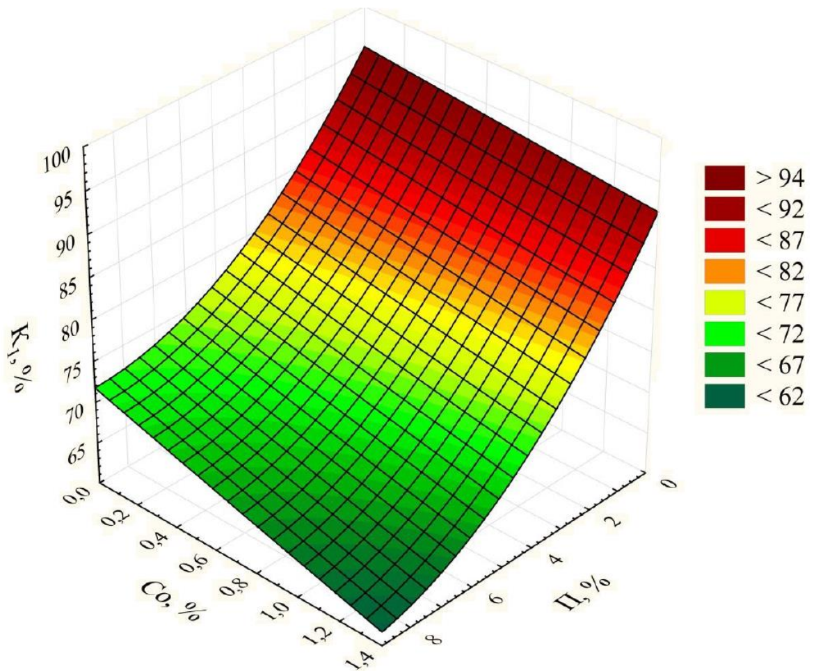
Рис. 3.9 – Залежність кількості насіння від складу вихідного вороху: K_1 – частка (кількість) насінневої фракції від вихідного вороху (вихід насіння), %; \Pi – вміст домішок у вихідній купі, %; C_0 – вміст обвалених зернівок гречки на вихідному купі, %
