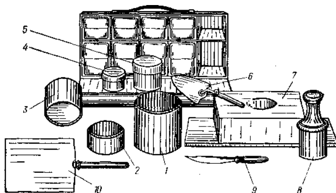
Мал. 2. Прилад Качинського для визначення об'ємної маси ґрунту.
