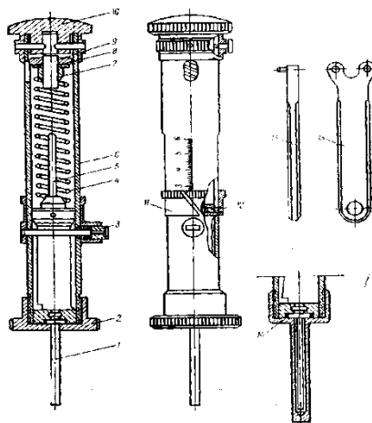
Мал. 7. Твердомір Качинського.
