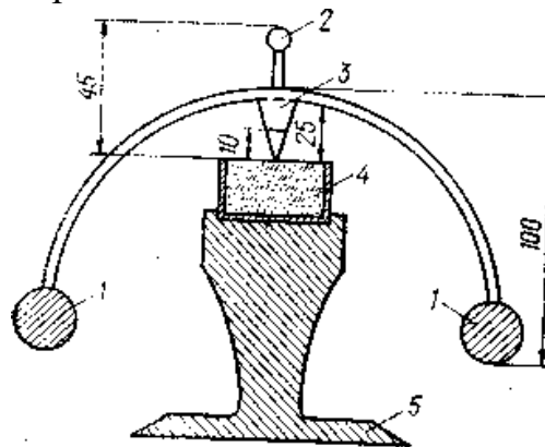
Мал. 5. Балансирний конус Васильєва
