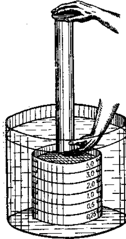
Мал. 3. Мокре просіювання за методом Саввінова
