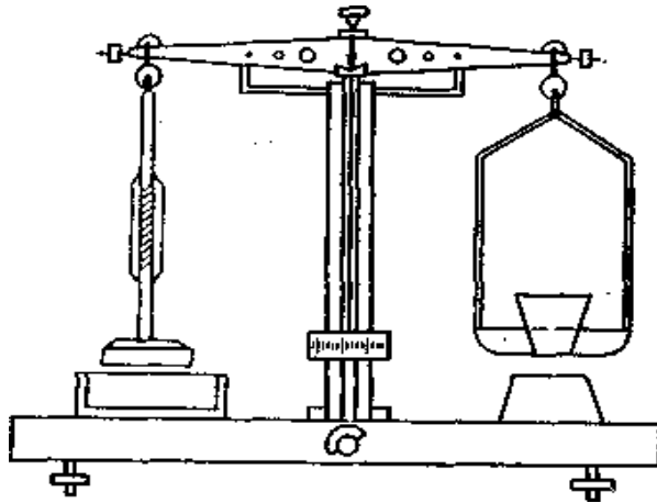
Мал. 6. Прилад Качинського для визначення липкості ґрунту
