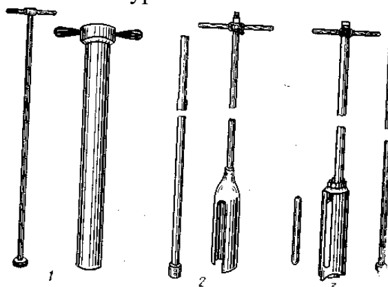
Мал.2. Бури для відбирання зразків ґрунту на вологість: 1 – бур Качинського, 2 – бур Ізмаїльського, 3 – бур Некрасова.
