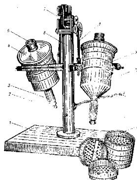
Мал. 4. Прилад Бакшеєва для агрегатного аналізу
