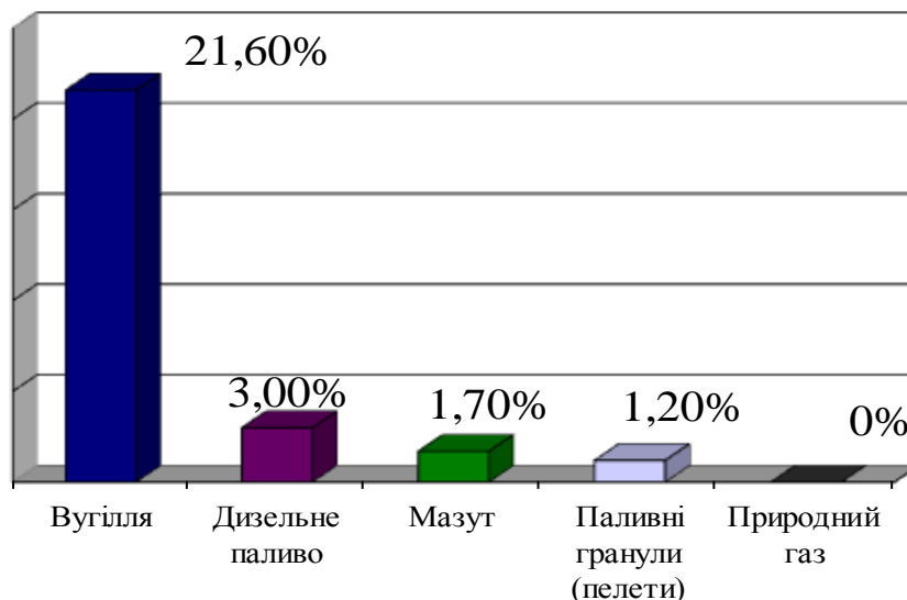
Рис. 3.2. Вміст золи у викидах при спалюванні різних видів палива, %.
