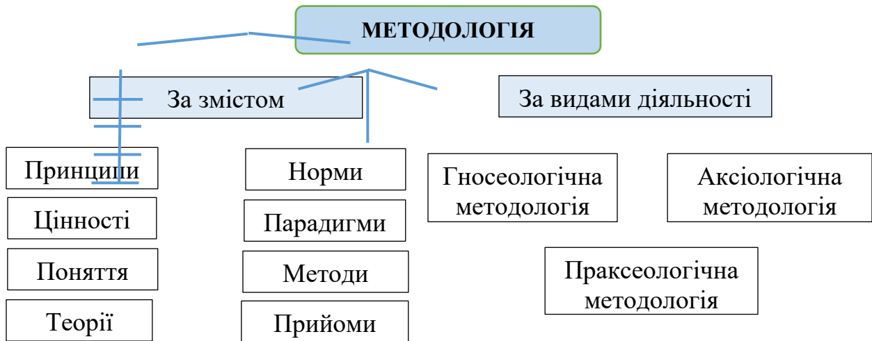
Рис. 4.1. Структура методології
