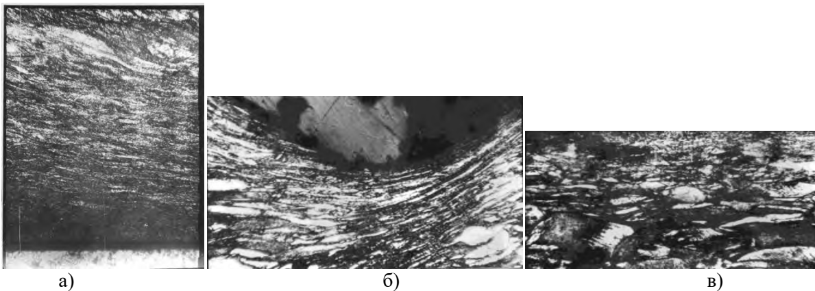
Рис. 5. Вид мікроструктури мідної заготовки в характерних точках сформованого профілю відповідно до рис. 5а: а) – точка 1 (зона контакту з валком); б) – точка 2; в) – точка 3
