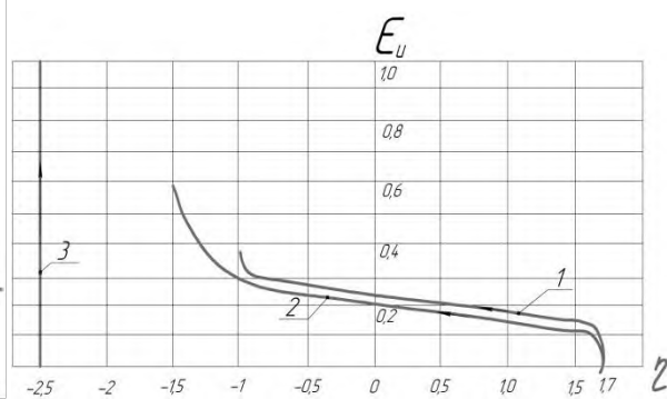
Рис. 9. Шляхи деформування часток матеріалу заготовки в найбільш деформованих зонах: 1 – посередині бічної поверхні АС; 2 – на вході в формотворюючий канал (поблизу точки А); 3 – в зоні контакту заготовки з валком
