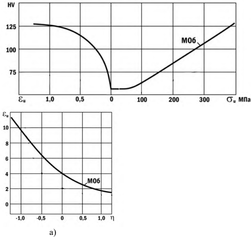
Рис. 6. Механічні характеристики міді М06: а) градувальний графік ( \sigma_u - HV - \varepsilon_u ); б) діаграма пластичності \varepsilon_u = \varepsilon_u(\eta) . HV – твердість по Віккерсу,
