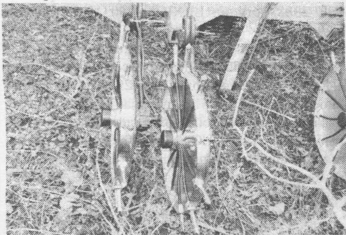
Рисунок - Инъекционные рабочие органы SpikeWheel
