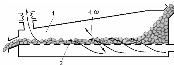
Рис. 2. Принципиальная схема вибротранспортера
