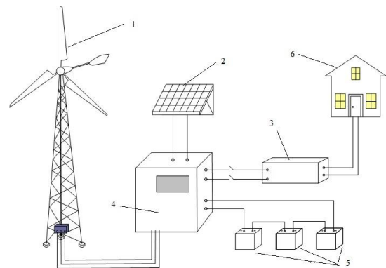
Рис. 4. Схема вітро-сонячної гібридної установки
