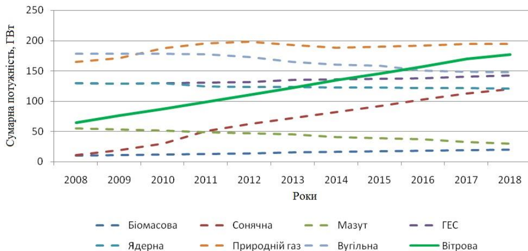
Рис. 1. Сумарна потужність електрогенерації в ЄС 2008-2018 рр.
