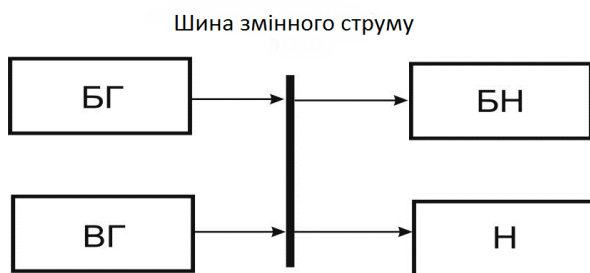
Рис. 5. Гібридна система автономного електропостачання: БГ – бензиновий електрогенератор; ВГ – вітровий генератор; БН – баластне навантаження; Н – навантаження
