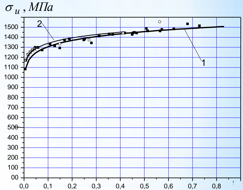
Крива течії сталі 30X3MФА після термообробки (крива 1 - стиск, крива 2 - розтяг).
