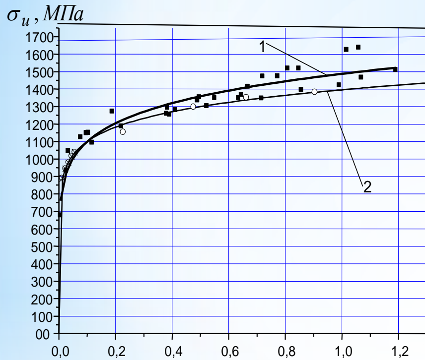
Крива течії сталі 38X2MЮА (крива 1 - стиск, крива 2 - розтяг)
