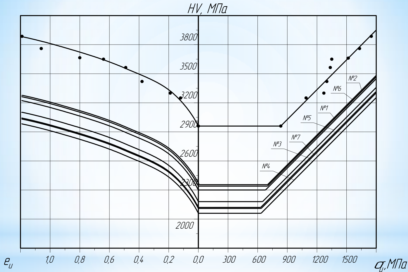
Градуювальні графіки сталі 38Х2МЮА після термообробки для семи досліджуваних зразків
