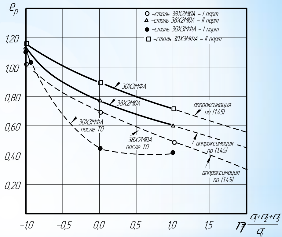
Діаграми пластичності сталей 30X3MFA і 38X2MЮA в стані поставки і після термообробки
