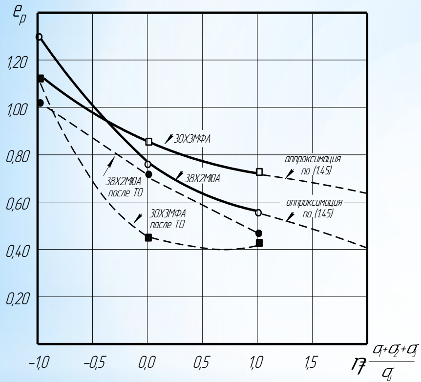
Діаграми пластичності сталей 30X3MFA і 38X2MЮA в стані поставки і після термообробки
