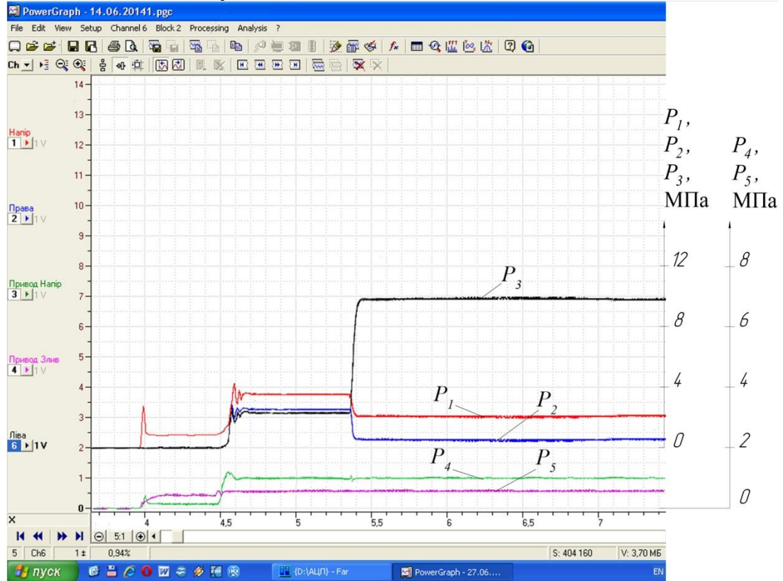
Рис. 3. Осцилограма роботи системи рульового керування при швидкості обертання вхідного вала n_e=80 об/хв та дії попутного навантаження \Delta p_n = -10 МПа
