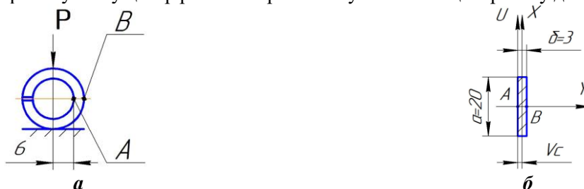
Рис. 4. Втулка розрізна: a – схема навантаження; b – переріз у критичних точках
