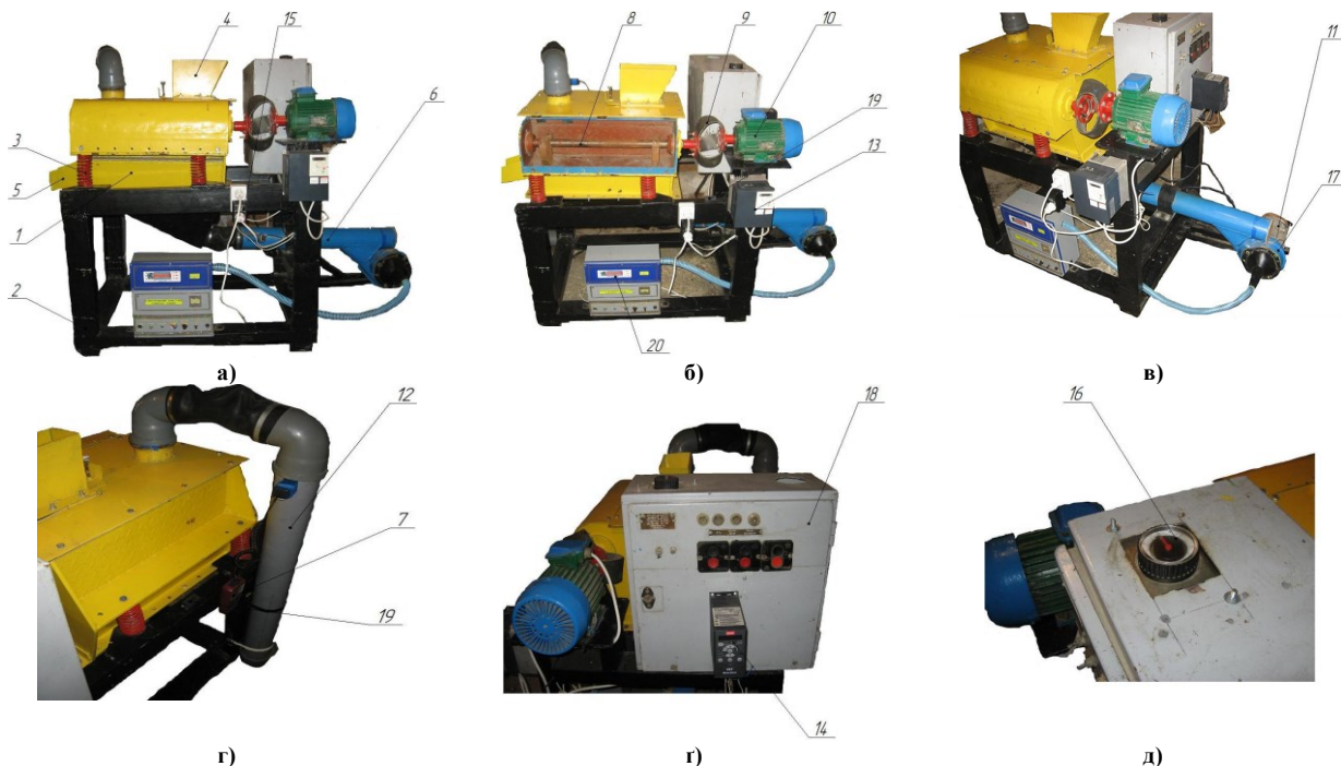
Рис. 1. Дослідна модель віброозонуючого комплексу: а), б) вигляд спереду; в), г), г) вигляд збоку; д) вигляд зверху; 1 – U-подібна камера; 2 – рама; 3 – пружини; 4, 5 – завантажувальний і розвантажувальний лотки; 6, 12 – відповідно вхідний та вихідний повітропроводи; 7 – термоанемометр; 8 – дебалансний вал; 9 – еластична муфта; 10 – електродвигун привода дебалансного вала; 11 – електродвигун привода вентилятора; 13, 14 – частотні перетворювачі; 15 – терморегулятор; 16 – реле часу; 17 – вентилятор; 18 – блок керування; 19 – вологоміри; 20 – електронний пристрій синтезу озону
