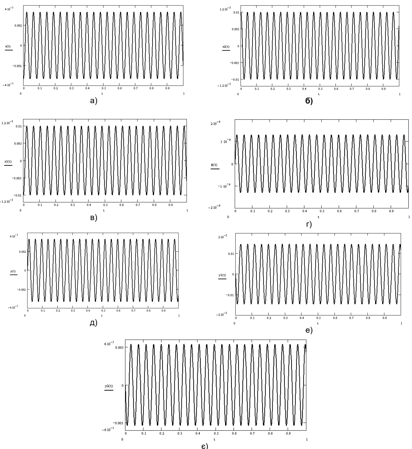
Рис. 1. Графіки функцій – рішень системи диференціальних рівнянь (3), що відповідає сталим змушеним коливанням: а) x = f(t) ; б) x_1 = f(t) ; в) x_2 = f(t) ; г) \varphi = f(t) ; д) y = f(t) ; е) y_1 = f(t) ; є) y_2 = f(t)
