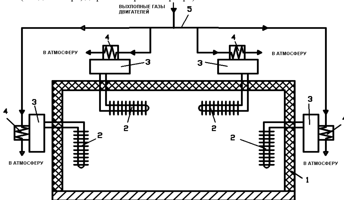
1 — холодильна камера; 2 — випарники АХА; 3 — теплорозсіюючі елементи АХА; 4 — кип'ятильник; 5 — магістраль підведення тепла
