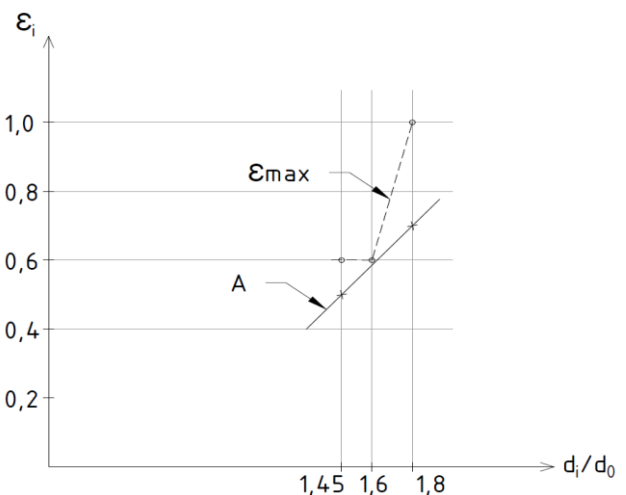
Рис. 6. Характер зміни інтенсивності деформацій на вільній зовнішній поверхні фланця (А) і в зоні максимальних деформацій \varepsilon_{max} у залежності від співвідношення діаметра фланця і вихідної заготовки
