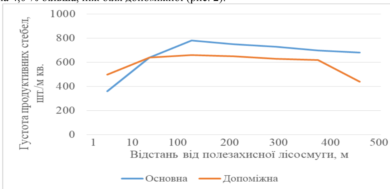
Рис. 1. Динаміка продуктивних стебел посівів пшениці озимої залежно від відстані від основної та допоміжної полезахисної лісосмуги
